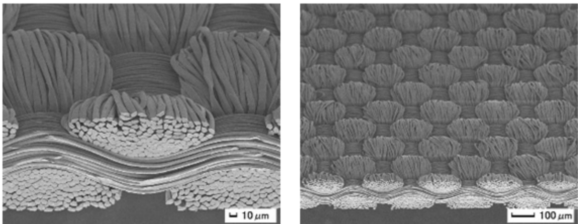
<그림 1> DELTA 2000의 단면사진
