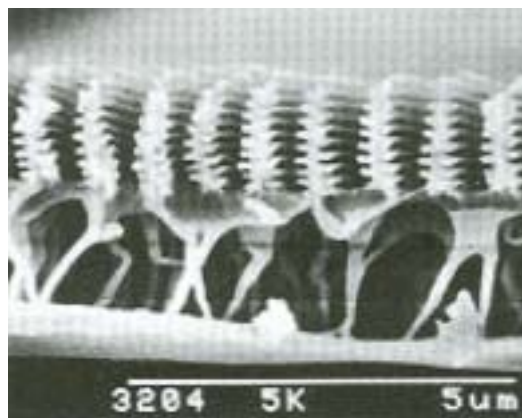
< 4> SEM
