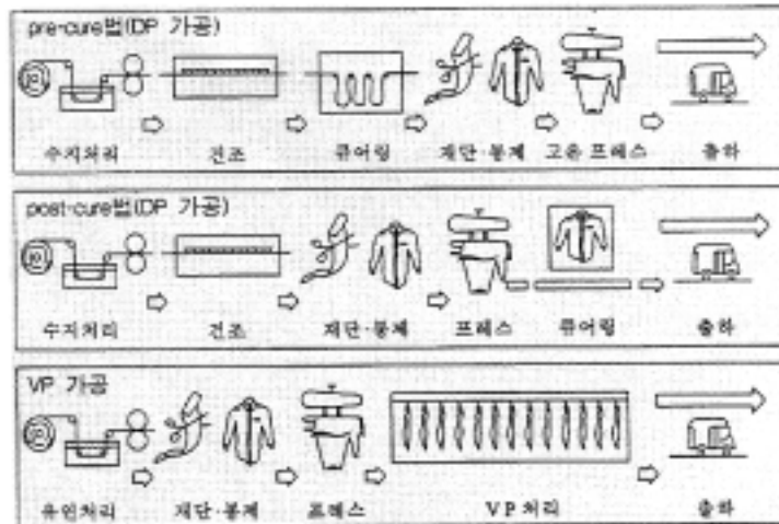
<그림> 재래식 DP 가공과 VP 가공 공정 비교
