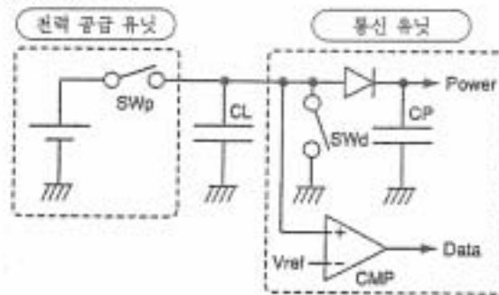
(C)등가 회로
