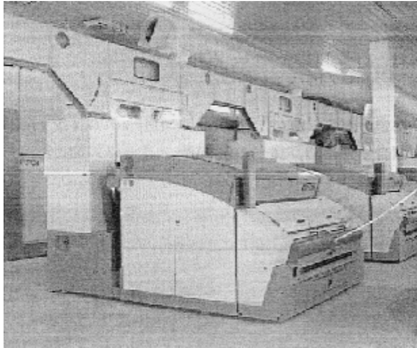
< 5> Rieter C60
