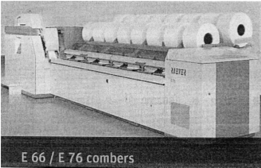
< 6> Rieter E66/E76( )
