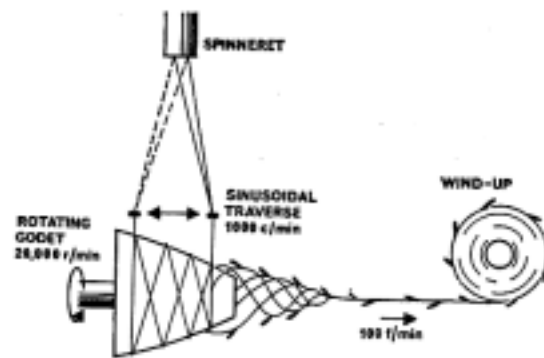
Fig. 3 Godet-spinning
