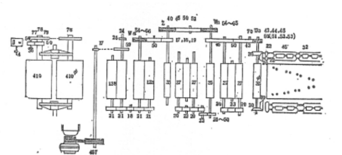
< 1-4> SLM E2/4 Gearing Diagram( )
