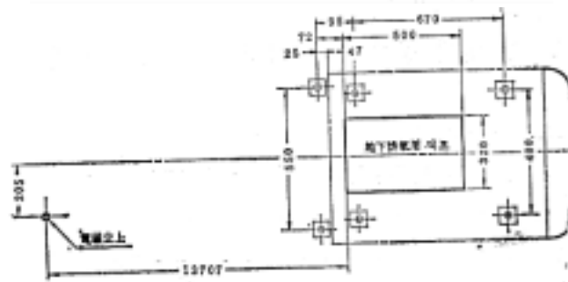
지하배기 덕트용 도면
