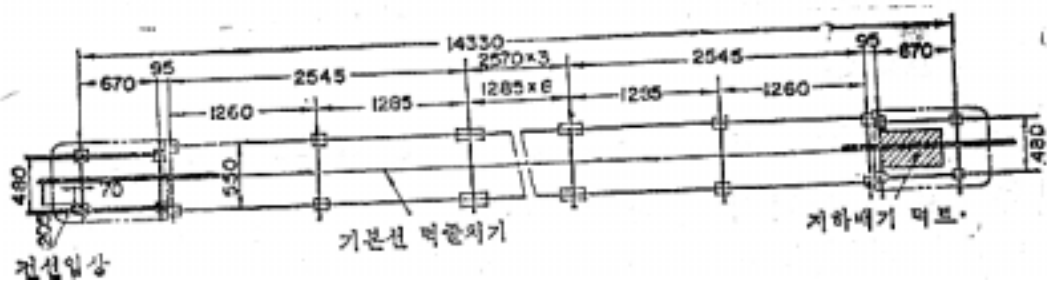
지하배기 덕트용 도면
