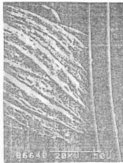
(나) 결점부 확대 (×800)
